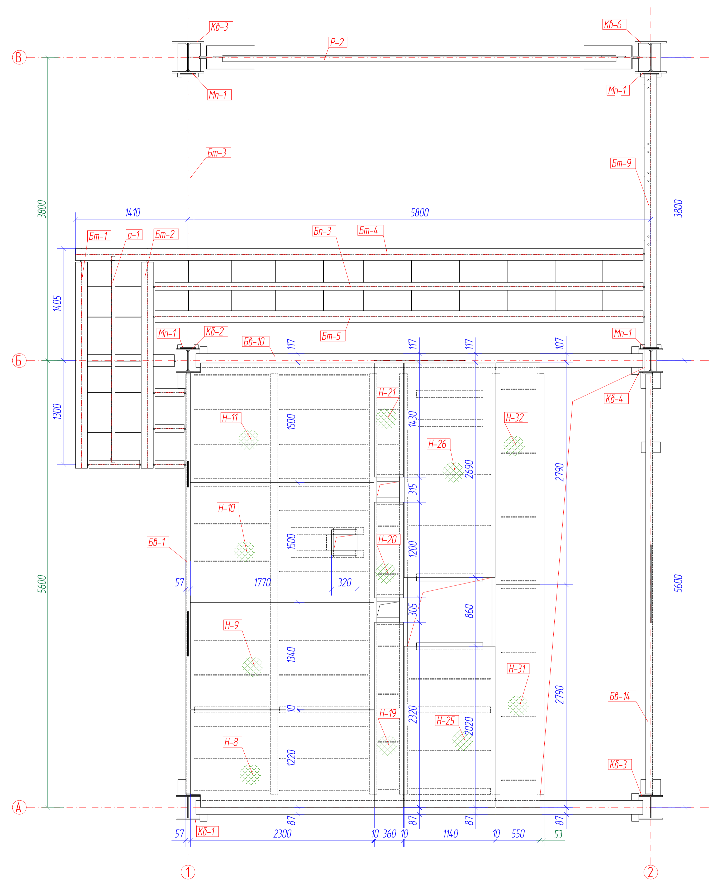
Схема расположения настила на отм. +25,700
