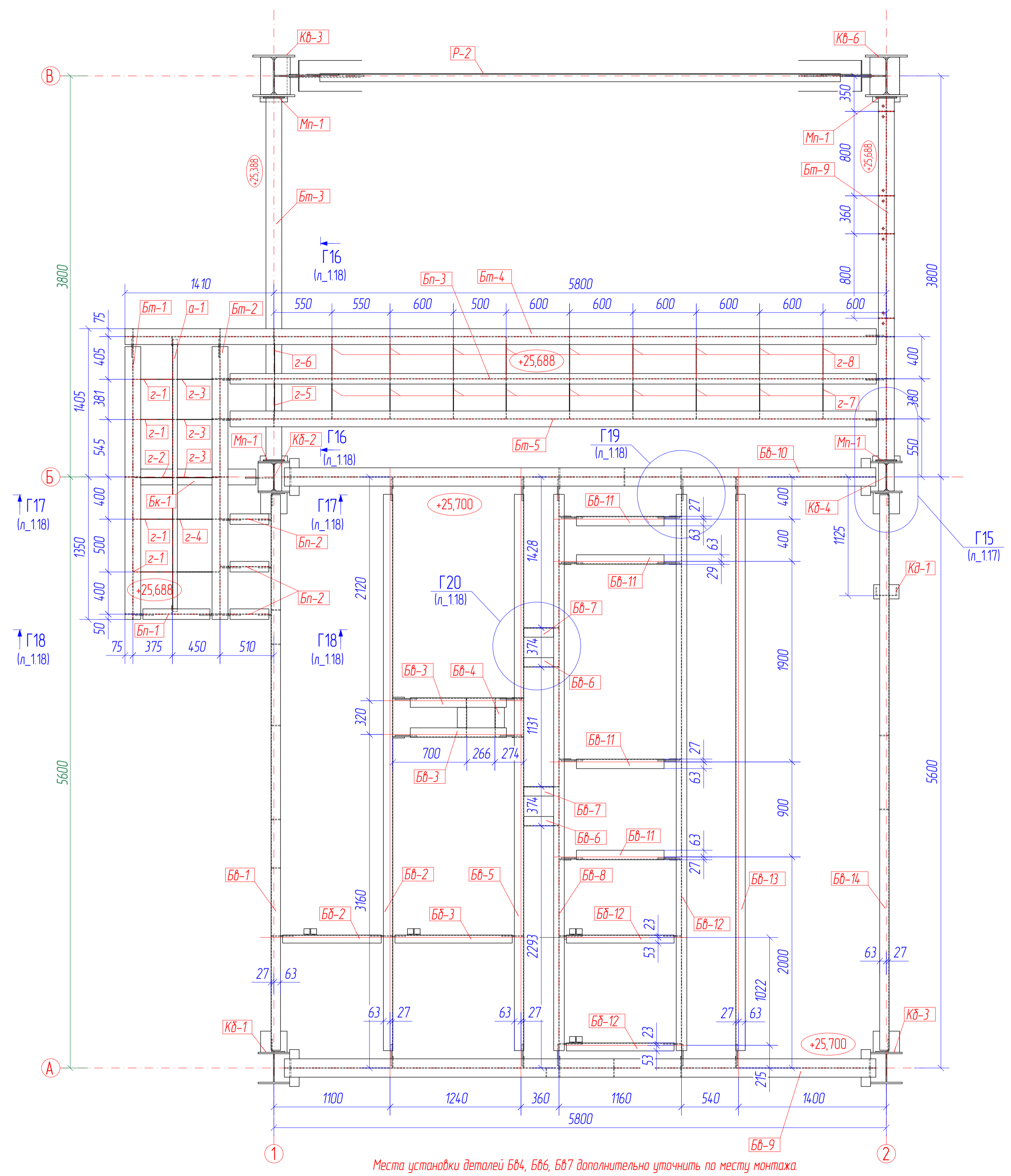
Схема расположения балок на отм. +25,700 (настил условно не показан)
