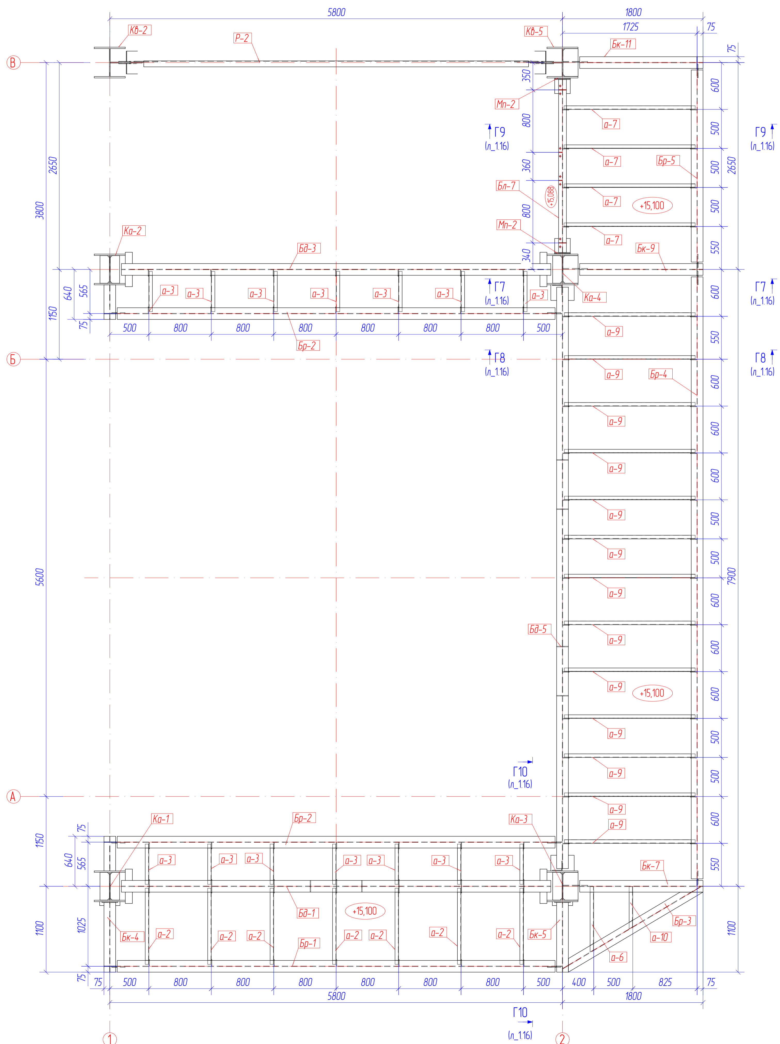
Схема расположения балок площадки на отм. +15,100
