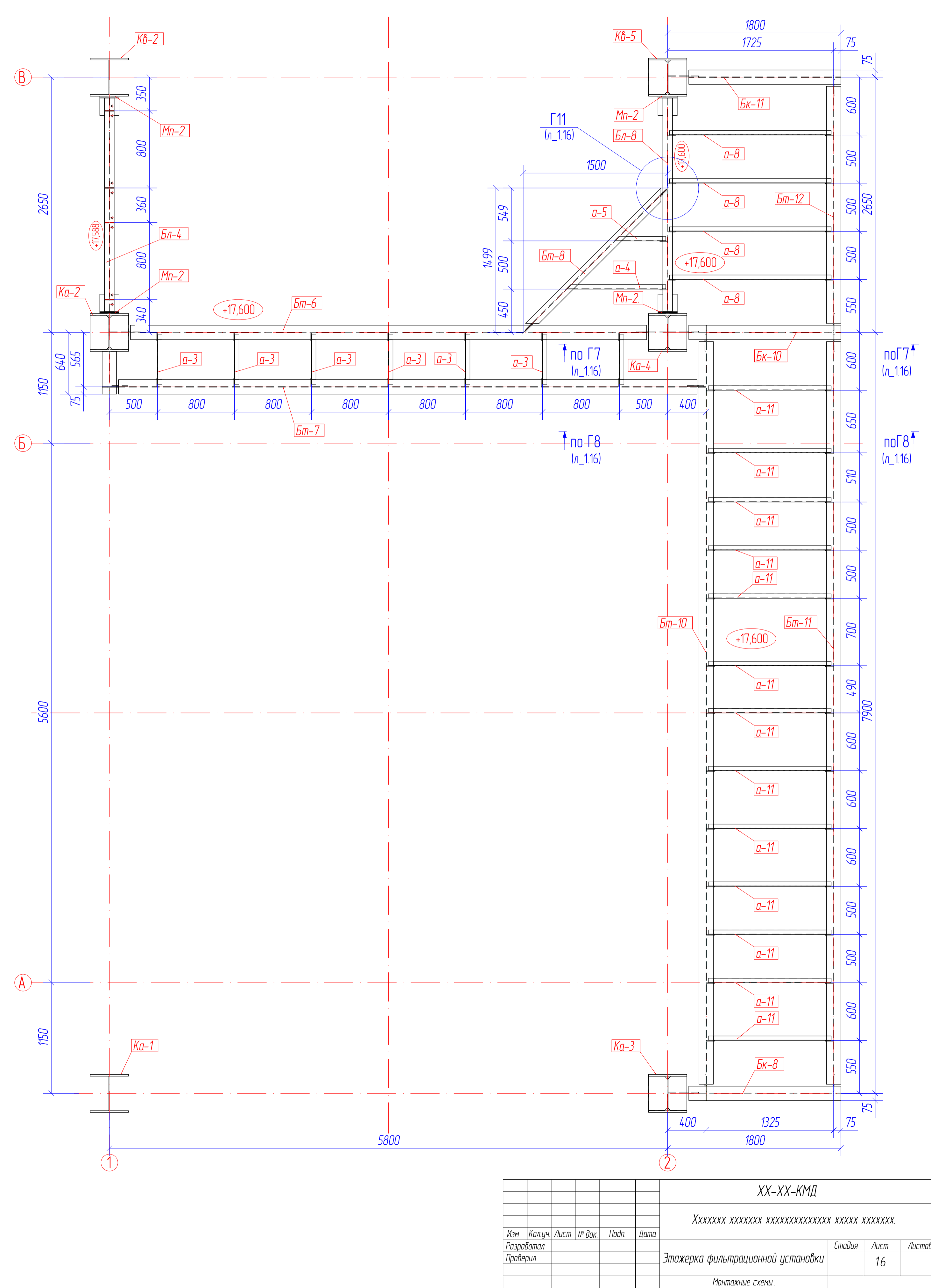
Схема расположения балок площадки на отм. +17,600
