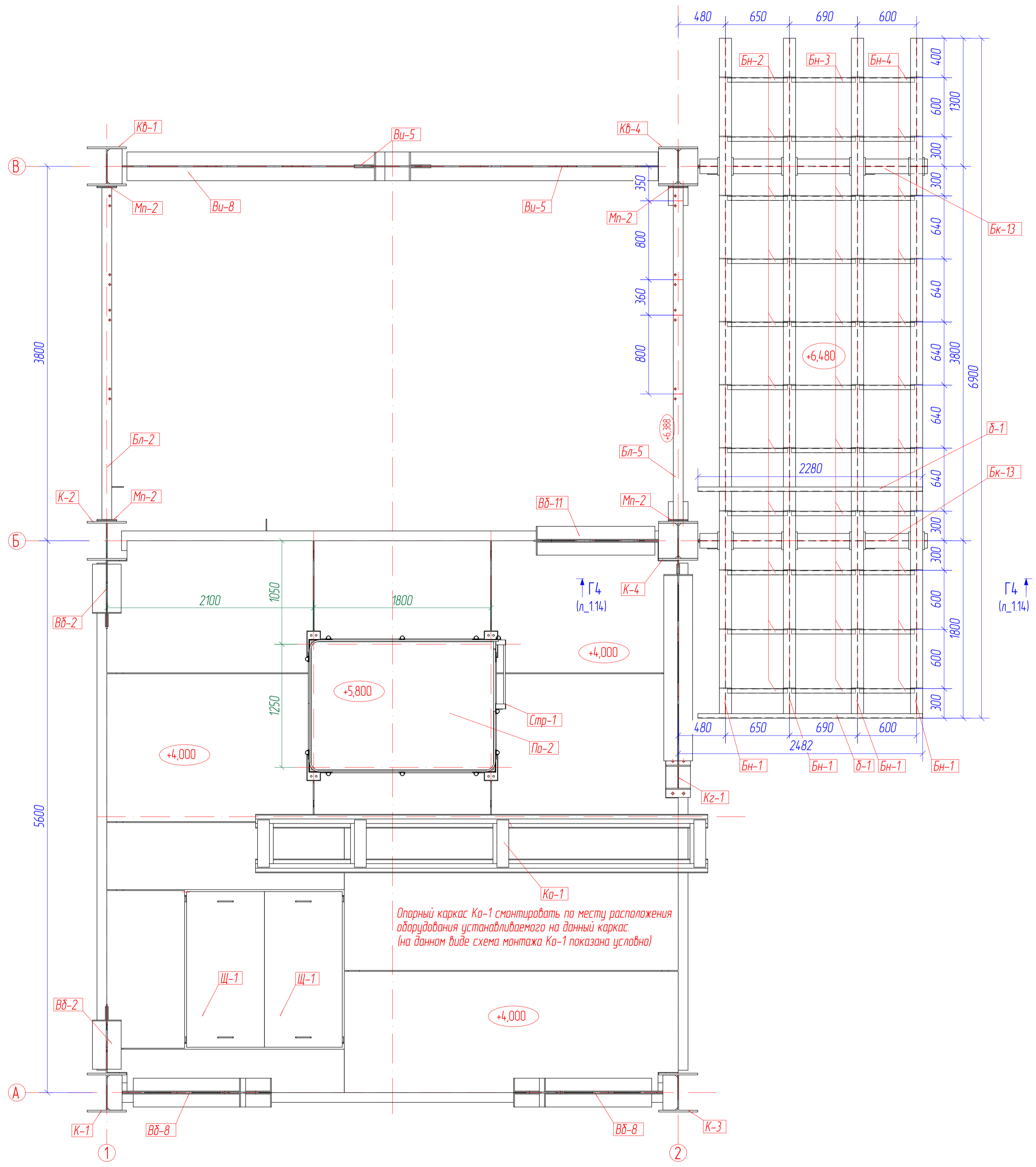
Схема расположения балок площадки на отм. +6,480
